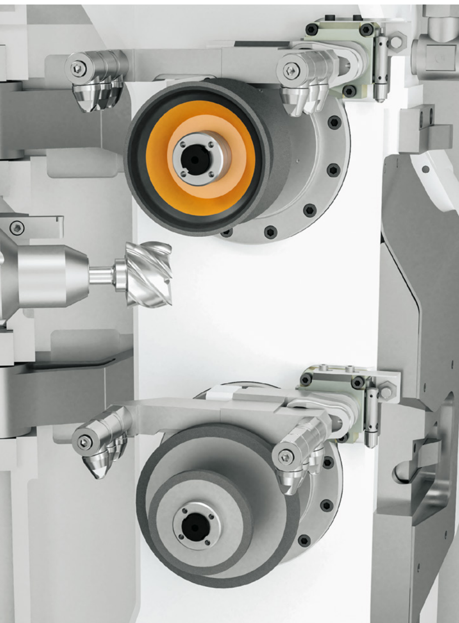
//////// Hybrid 260 mit einem neuen und innovativen Maschinenkonzept
