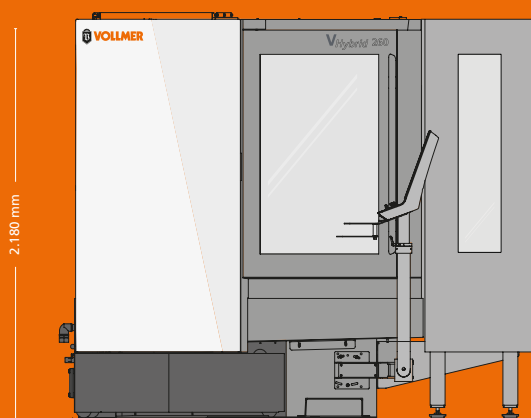
/////// MASCHINENABMESSUNGEN VHybrid 260 mit HC 4
