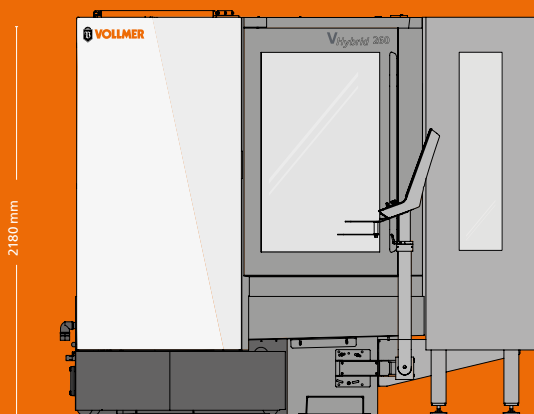
////// WYMIARY MASZINY VHybrid 260 z HC 4
