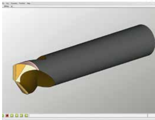
/////// SYMULACJA OPERACJI ERODOWANIA Erodowanie PCD
