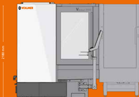
////// DIMENSIONES DE LA MÁQUINA VGrind 360S con HPR 250
