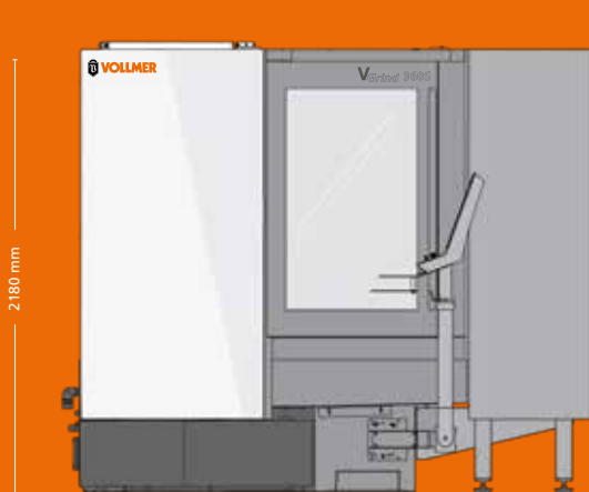
////// DIMENSIONES DE LA MÁQUINA VGrind 360S con HP 160 o HC 4
