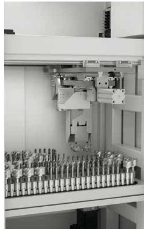
////// ALMACÉN DE CADENAS HC 4 para 39 herramientas HSK-A63 o hasta 158 herramientas de mango
